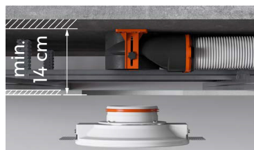
Minimální instalační výška: 140 mm ~ 5,51"
